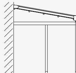
CONTRAVERSA E SOSTEGNO per strutture con profondità da 4,5 a 7,0 m (su richiesta)
